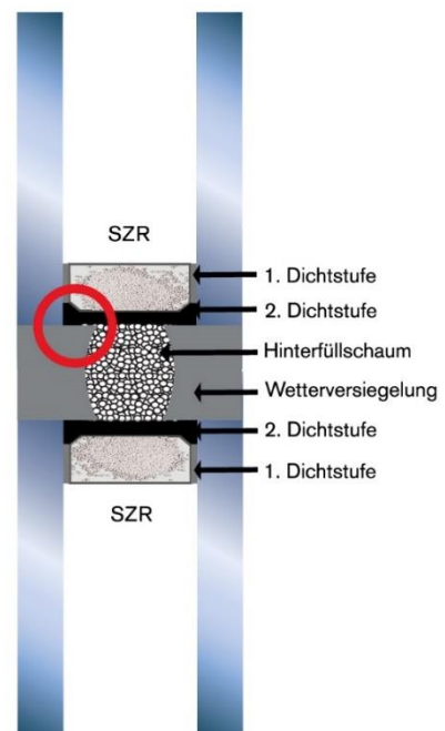
Wetterversiegelung in einem Isolierglasstoß
